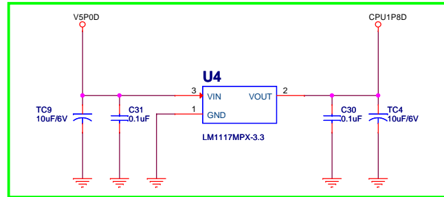
외부 LDO 사용시 R23 제거후 부품 장착
