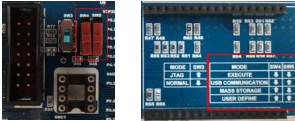
&lt;SW4, SW5 과 SW setting 방법&gt;
