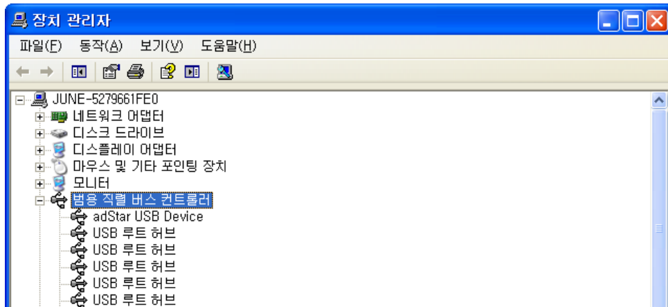
[ 장치관리자 ]
