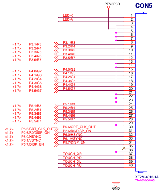
TM0520-0040 (상하접점)
